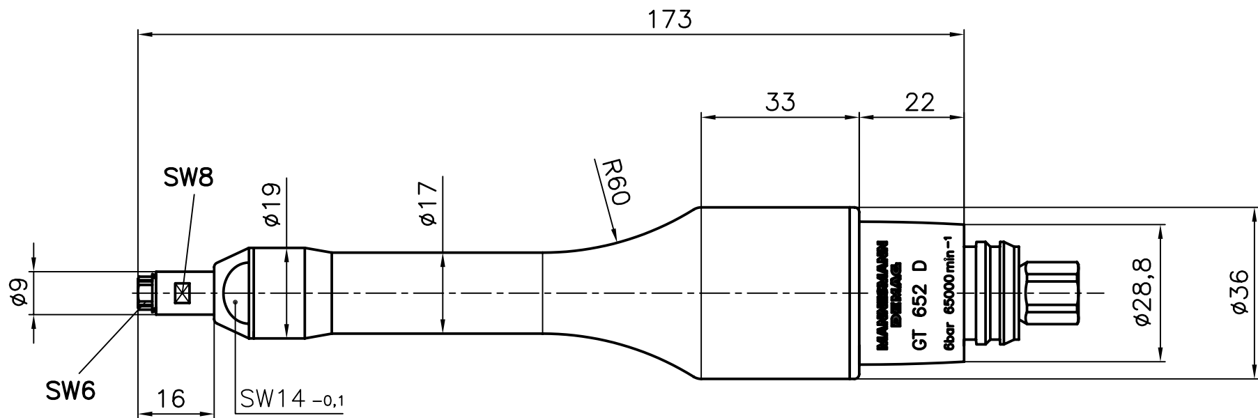
Turbinenschleifer GT 652 D 29940375
